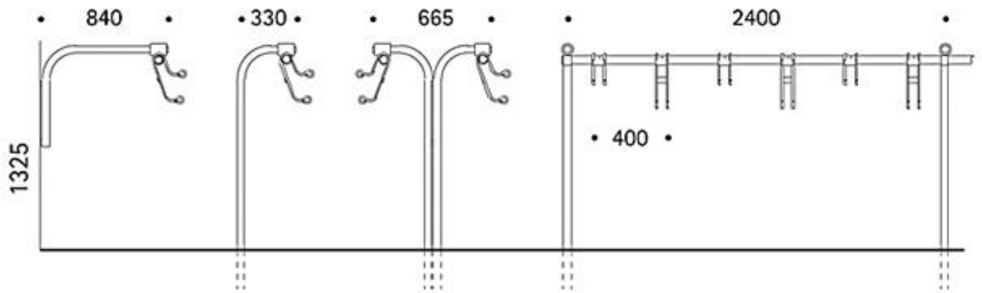
CC 240 V
